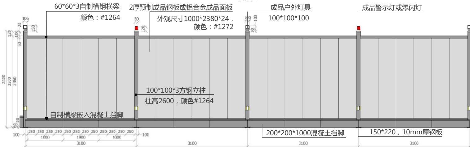
正视图
