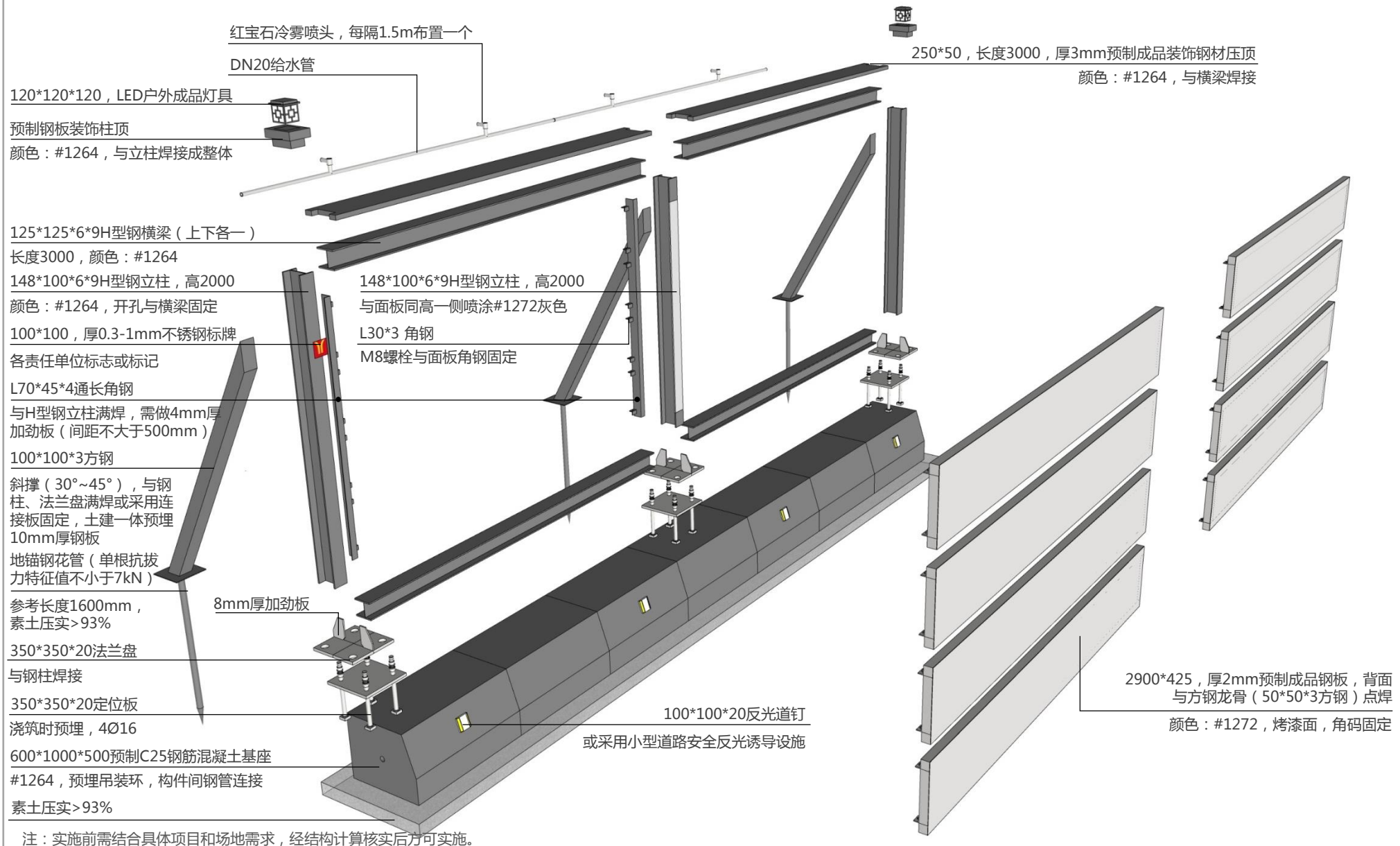
A2-1装配式H型钢结构围蔽一（结构一）拆分图
