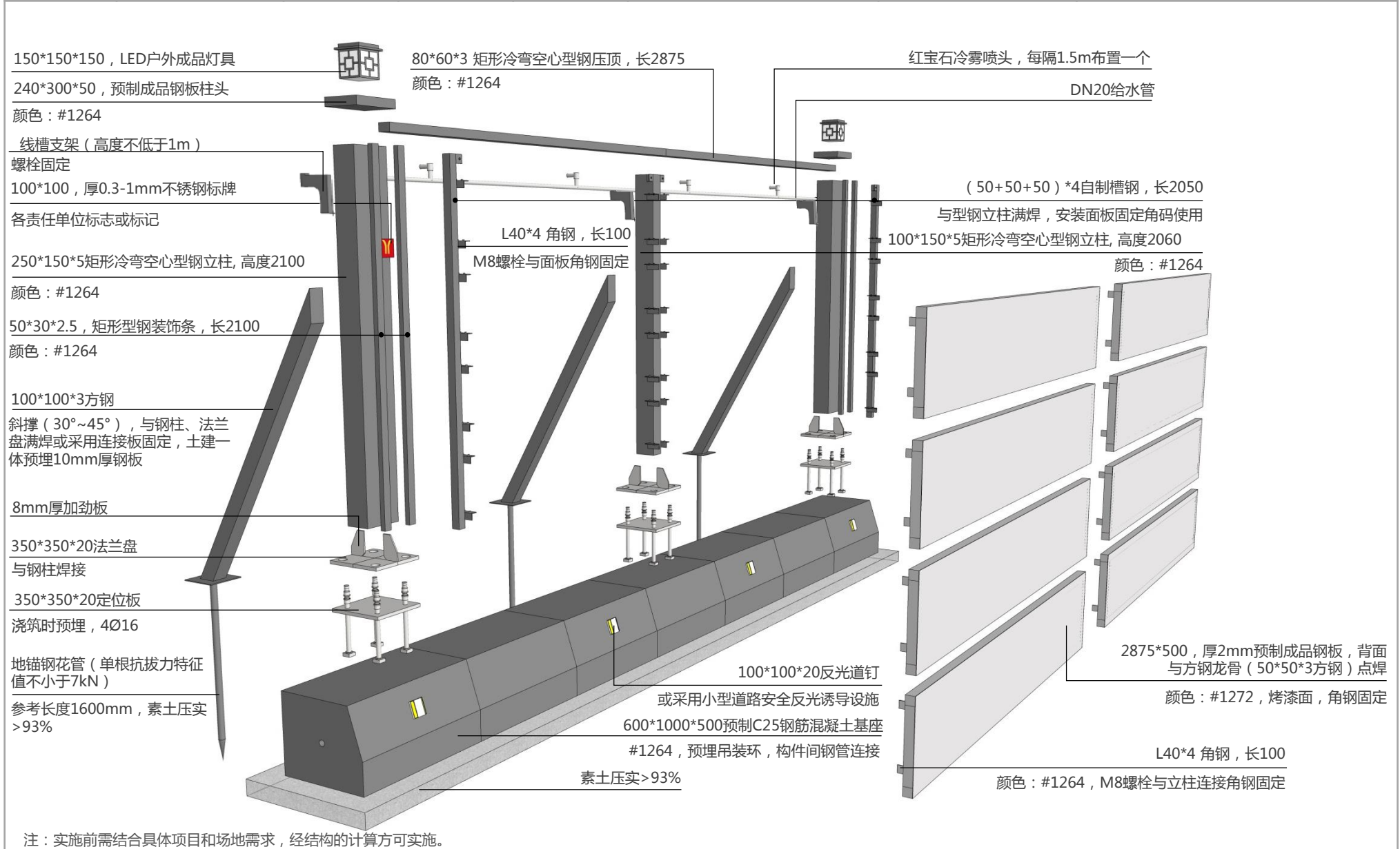
A1装配式方钢结构围蔽拆分图
