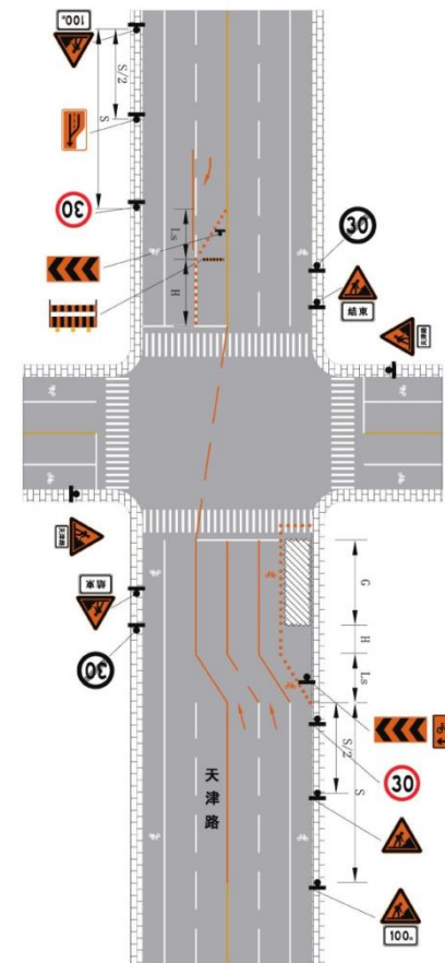
图 C.24 城市道路交叉口进口道作业区布置示例
