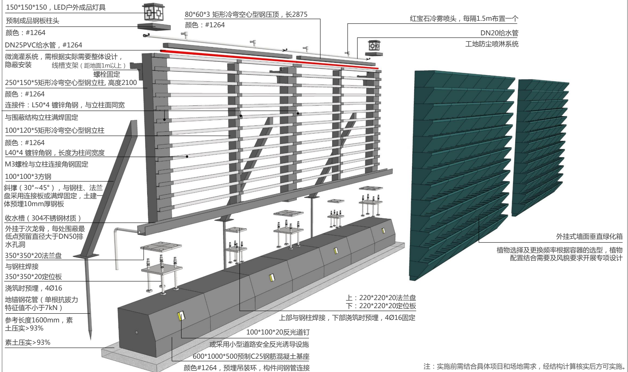
B1-1立体绿化围蔽拆分示意图 (基于A1型装配式方钢结构围蔽, 新建或改造的均可参考)
