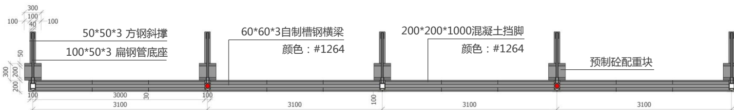
顶视图
