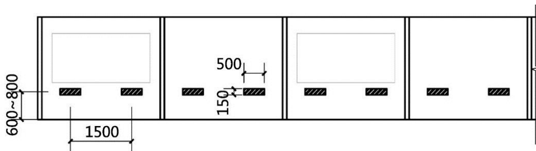
墙身反光标志（轮廓标）位置示意二
