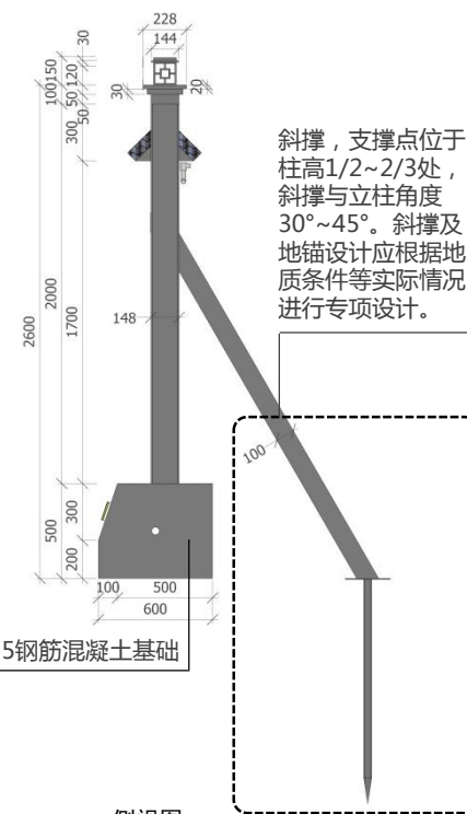
侧视图
