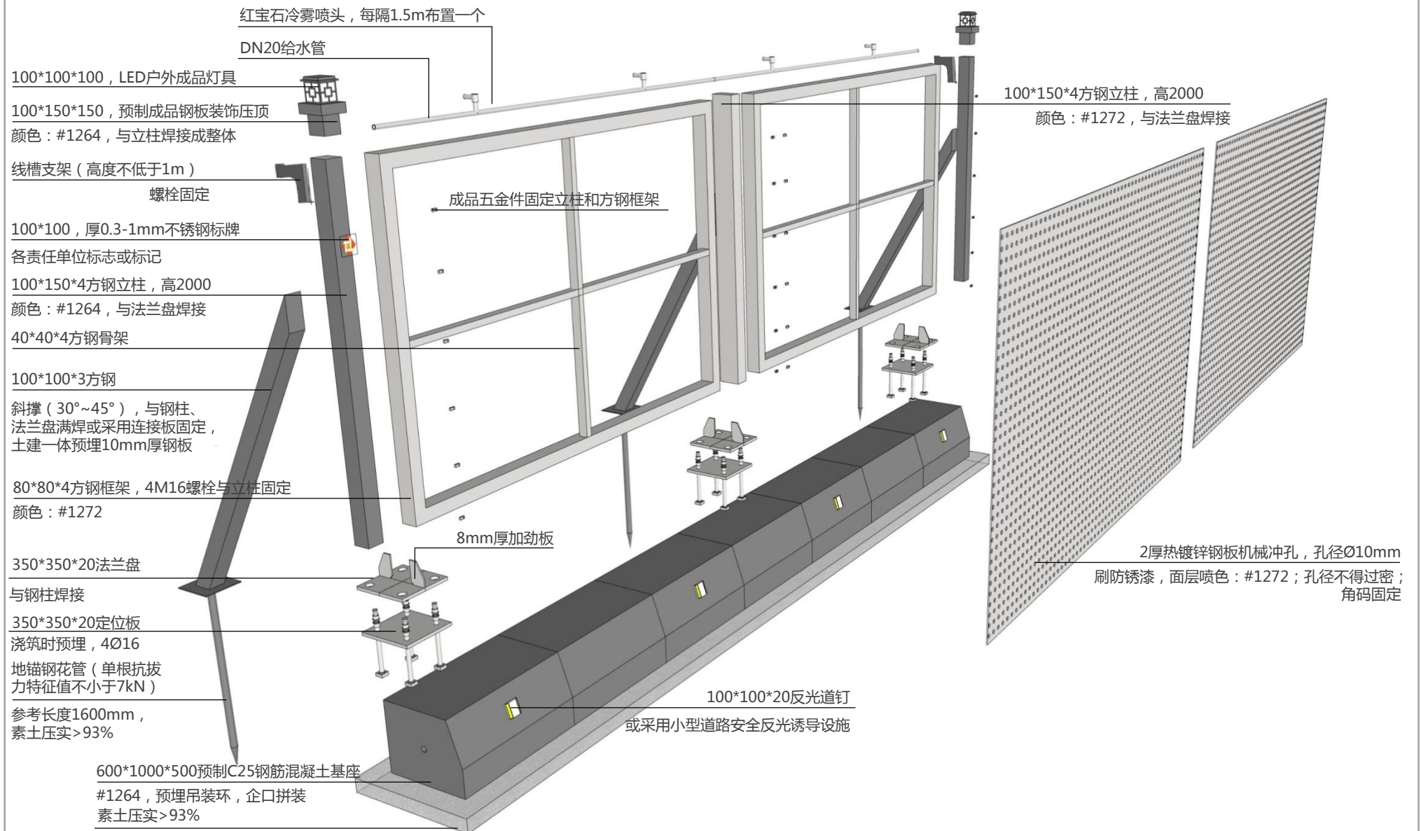
A4装配式穿孔金属板围蔽拆分图
